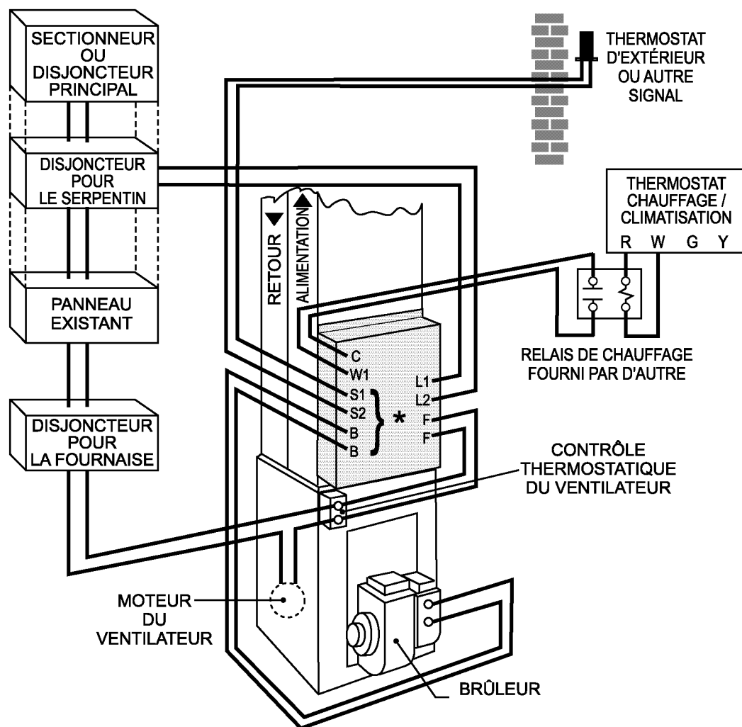
CÂBLAGE TYPIQUE APRÈS L'INSTALLATION DU SERPENTIN D'ADJONCTION
